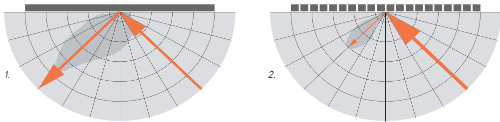
Diagramma di direttività di un'onda sonora incidente su superficie riflettente (1) e superficie assorbente (2).
