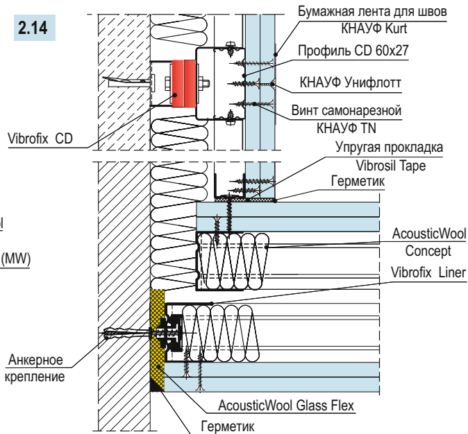
Горизонтальный разрез
